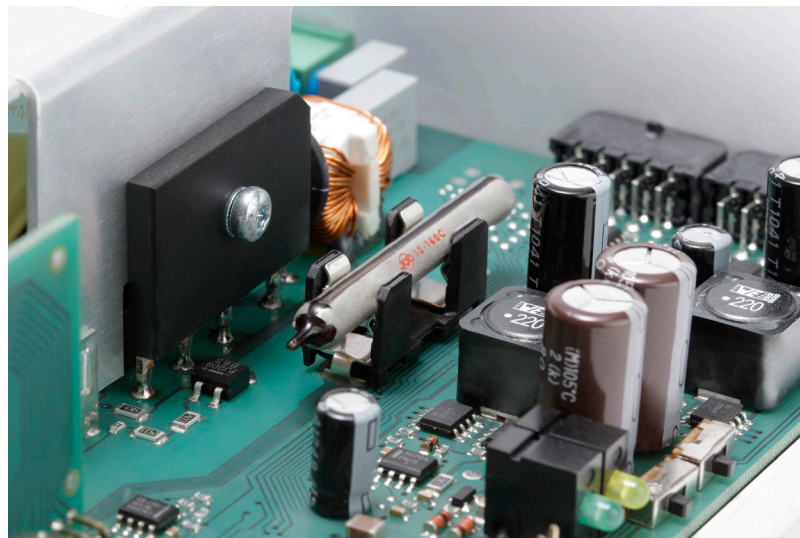
Innovative Löscheinrichtung zur Anwendung in elektrischen Geräten: Die E-Bulb® der Ahrensburger Firma JOB.
